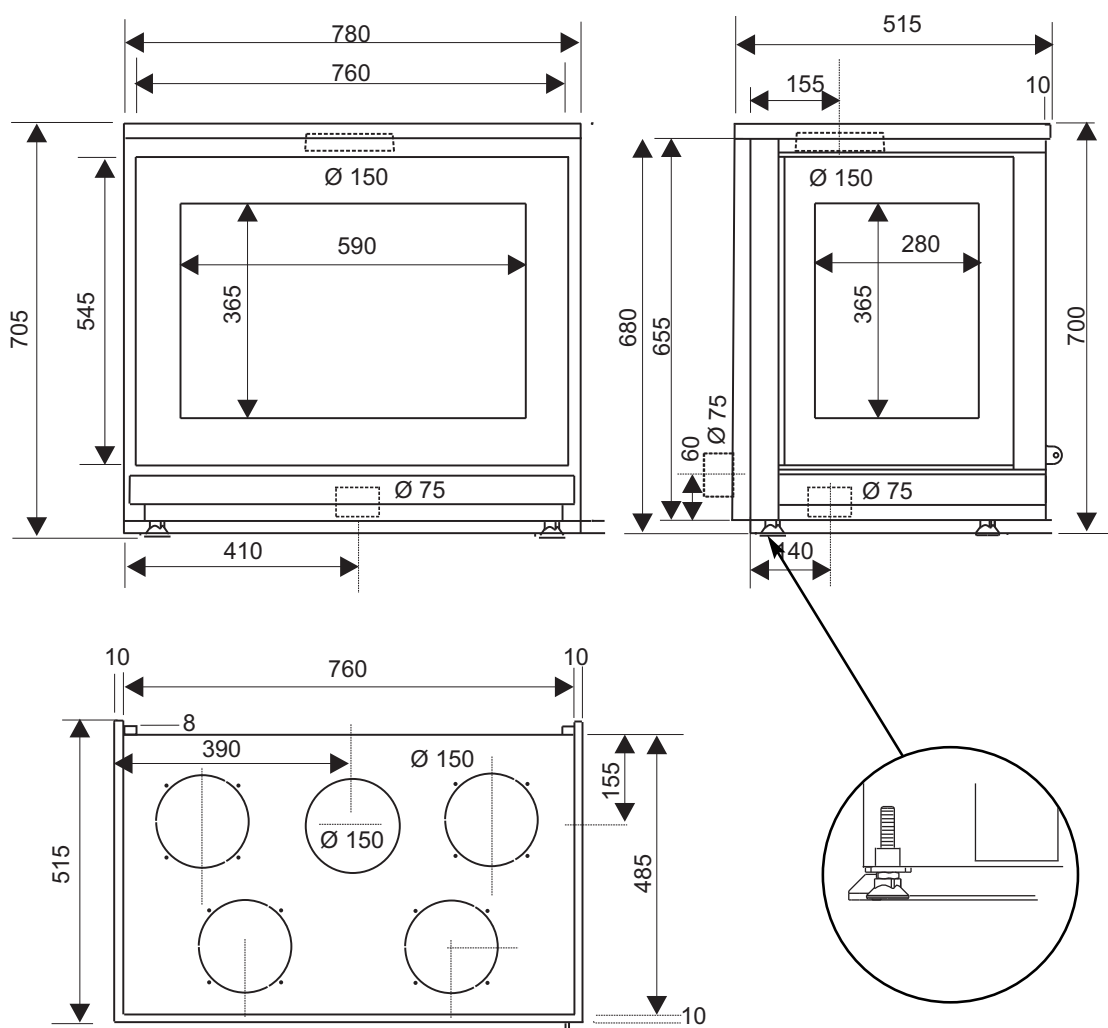
COTES NEO 76 VL2
