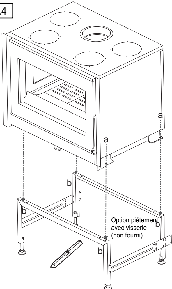
Principe de fixation du foyer sur le piétement PS 76 (option).
