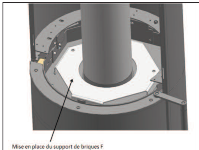
Support de briques F
